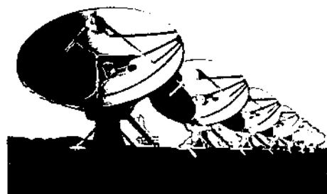
تلسکوپ رادیویی و بسیار بزرگ آرایه
