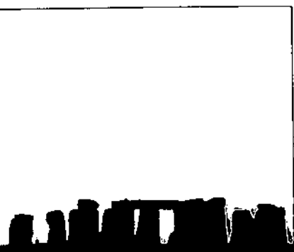
طلوع آفتاب در استون هیج
